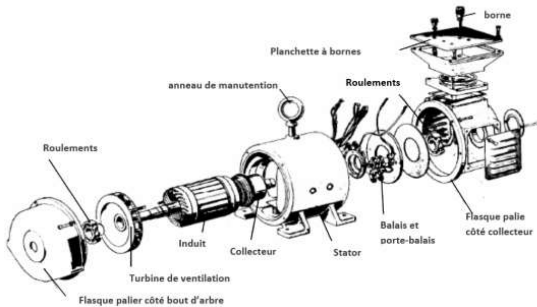
Fig 6 : Vue éclatée d'un moteur à courant continu
