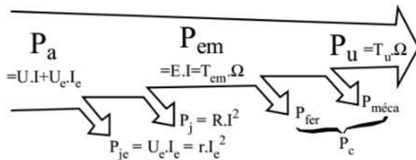
Fig 9 : Bilan de puissance du moteur c.c.
